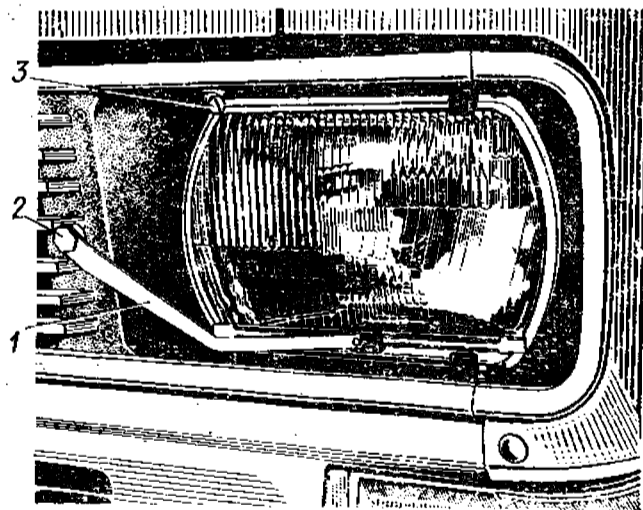
Рис. 85. Очиститель рассеивателей света фар:
