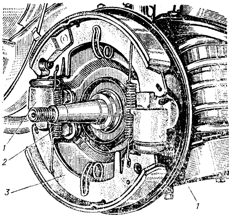
Рис. 76. Тормозной барабанный механизм переднего колеса:
