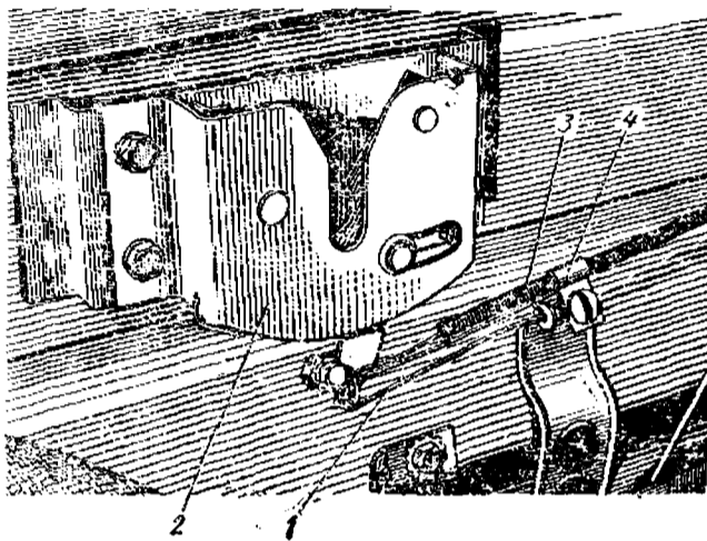
Рис. 14. Запор капота и его привод: 1 — аварийная тяга привода запора; 2 — запор капота; 3 — оболочка тяги привода запора; 4 — скоба, жестко закрепленная на оболочке
