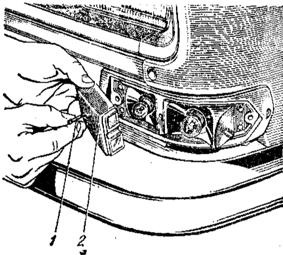
Рис. 89. Замена лампы в ручке выключателя аварийной сигнализации: 1 — контрольная лампа; 2 — ручка выключателя
