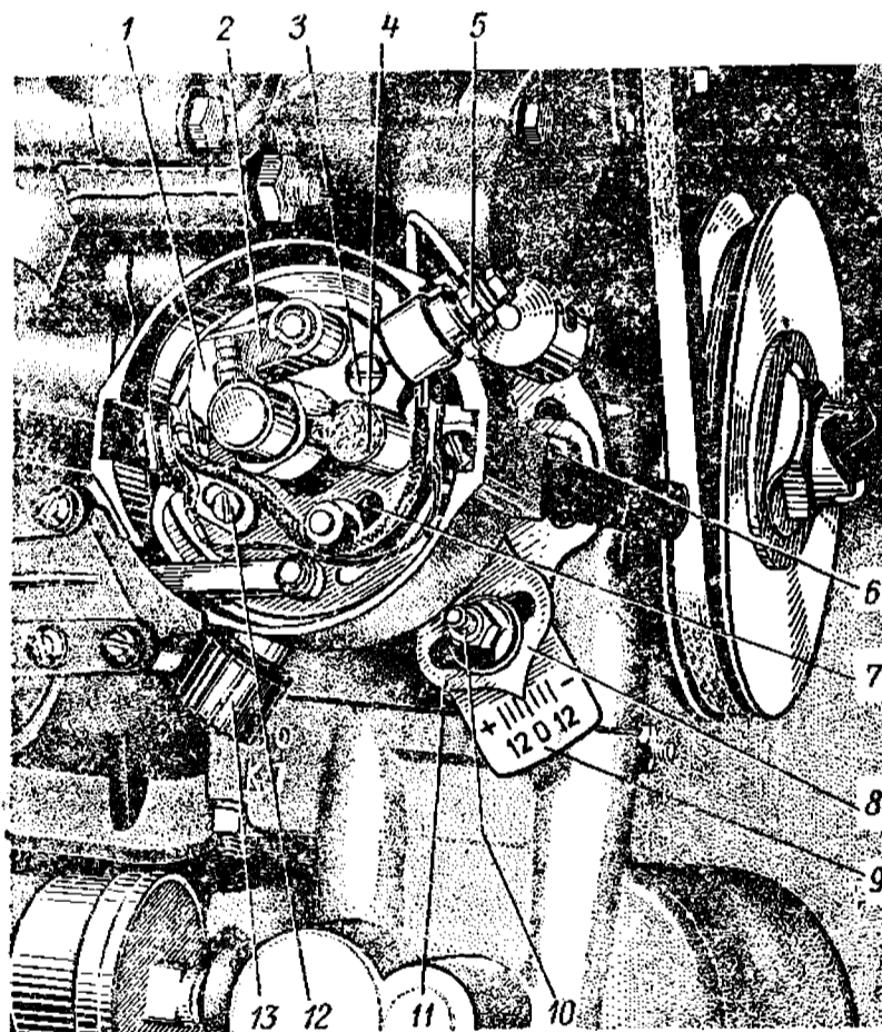
Рис. 81. Распределитель зажигания (со снятыми крышкой и ротором):
