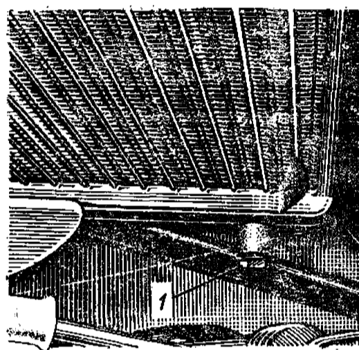
Рис. 37. Расположение пробки сливного отверстия на нижнем бачке радиатора:
