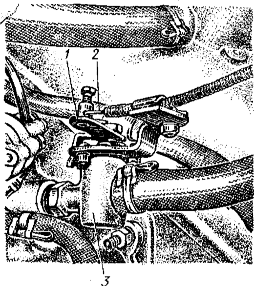
Рис. 36. Расположение крана отбора горячей жидкости из системы охлаждения в теплообменник отопителя кузова:
