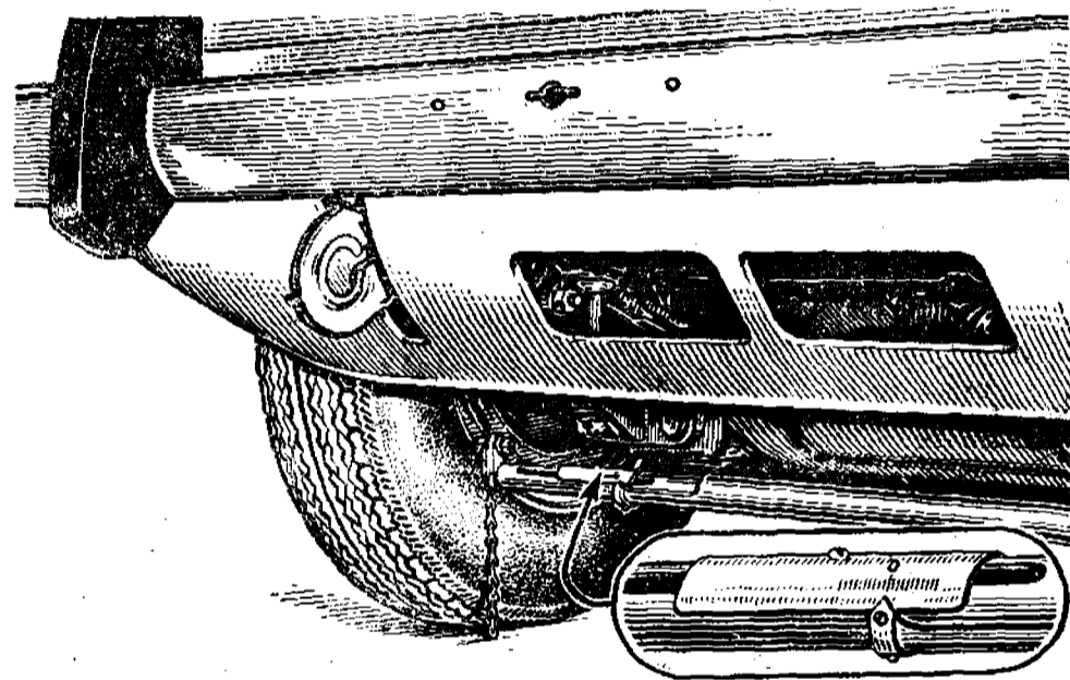
Рис. 70. Проверка раздвижной линейкой схождения передних колес
