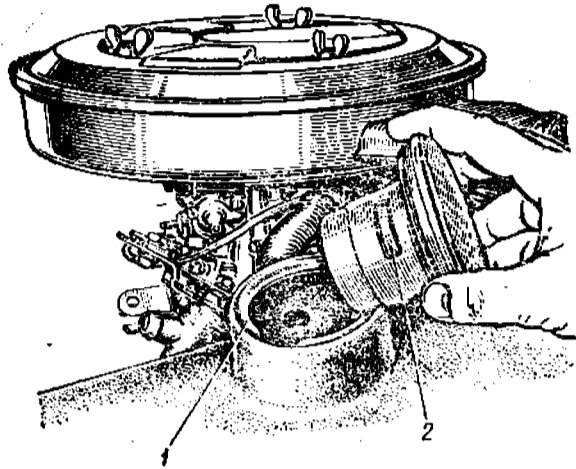
Рис. 42. Расположение маслonaполнительной горловины картера двигателя: 1 — горловина; 2 — фильтрующий элемент системы вентиляции картера
