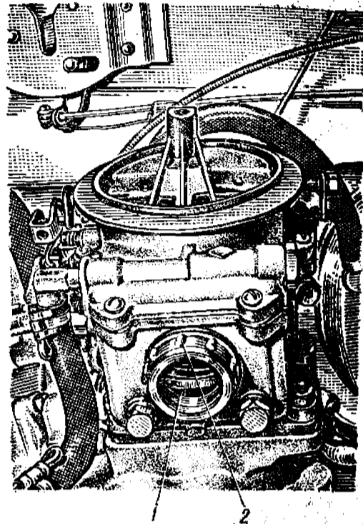
Рис. 60. Расположение смотрового окна на карбюраторе К-126Н: 1 — стекло; 2 — прижимная гайка
