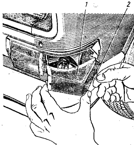
Рис. 89. Замена лампы в ручке выключателя аварийной сигнализации: 1 — контрольная лампа; 2 — ручка выключателя
