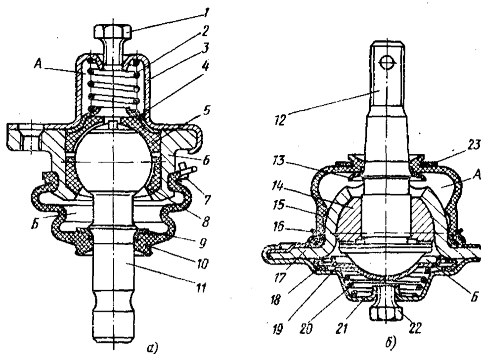
Рис. 73. Шаровые шарнир и опора стойки передней подвески:
