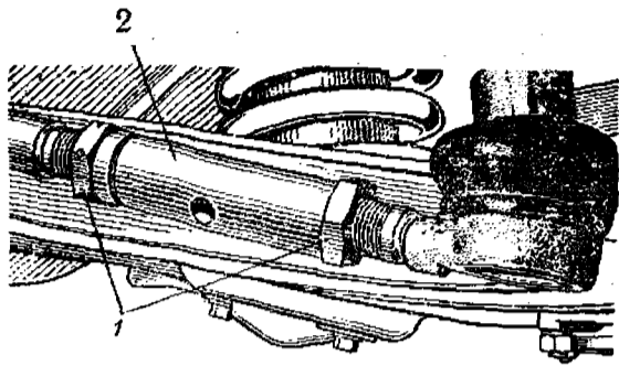
Рис. 71. Узел регулировки схождения передних колес:
