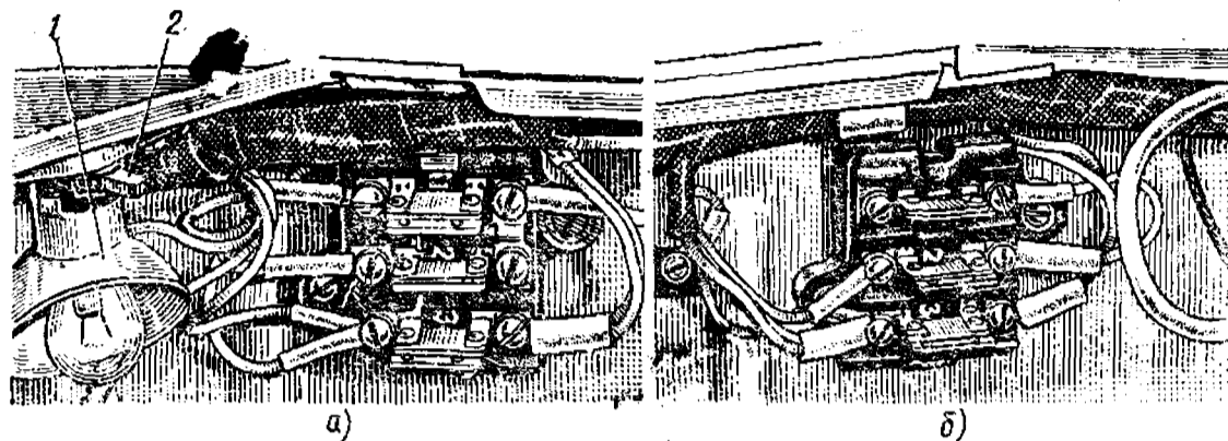
Рис. 83. Блоки плавких предохранителей (со снятыми крышками): а и б — блоки, установленные соответственно на левом и правом брызговиках передних крыльев; 1 — подкапотная лампа; 2 — выключатель лампы
