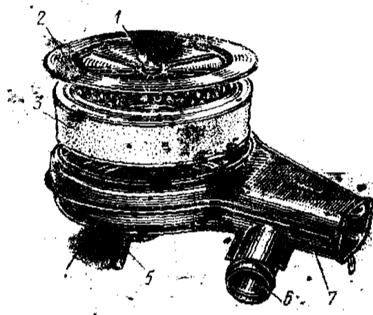
Рис. 64. Воздушный фильтр карбюратора К-126Н: 1 — барашковая шпилька; 2 — крышка корпуса; 3 — фильтрующий элемент; 4 — корпус; 5 — патрубок системы вентиляции картера; 6 — патрубок для подсоединения шланга подвода подогретого воздуха; 7 — входной патрубок корпуса
