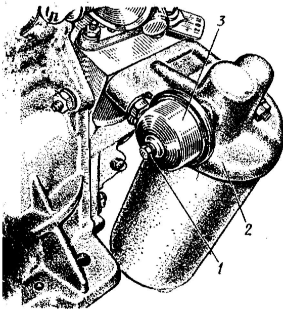
Рис. 45. Расположение датчика указателя давления масла:
