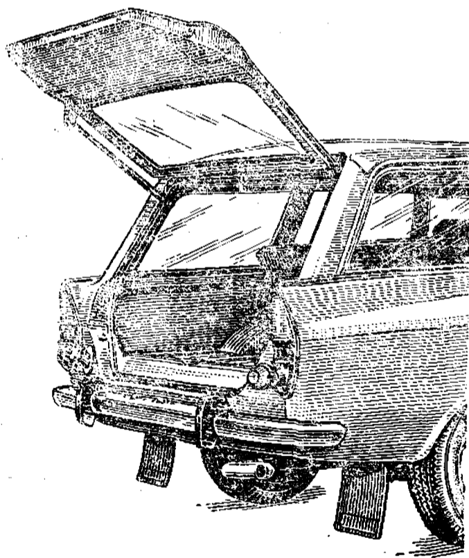
Рис. 4. Багажное отделение автомобиля «Москвич-1500» мод. 2137
