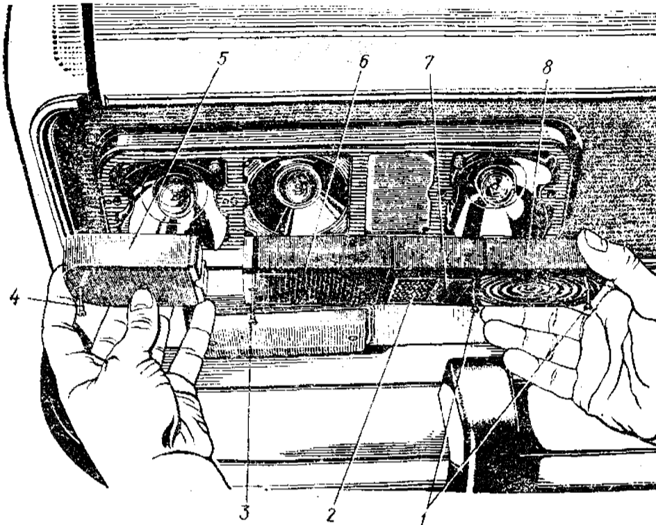
Рис. 92. Замена ламп в заднем комбинированном фонаре:
