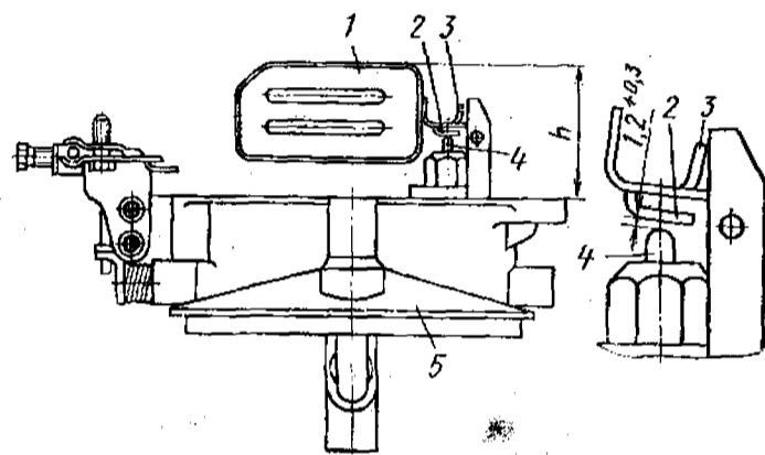
Рис. 61. Проверка установки поплавка на крышке поплавковой камеры карбюратора К-126Н:
