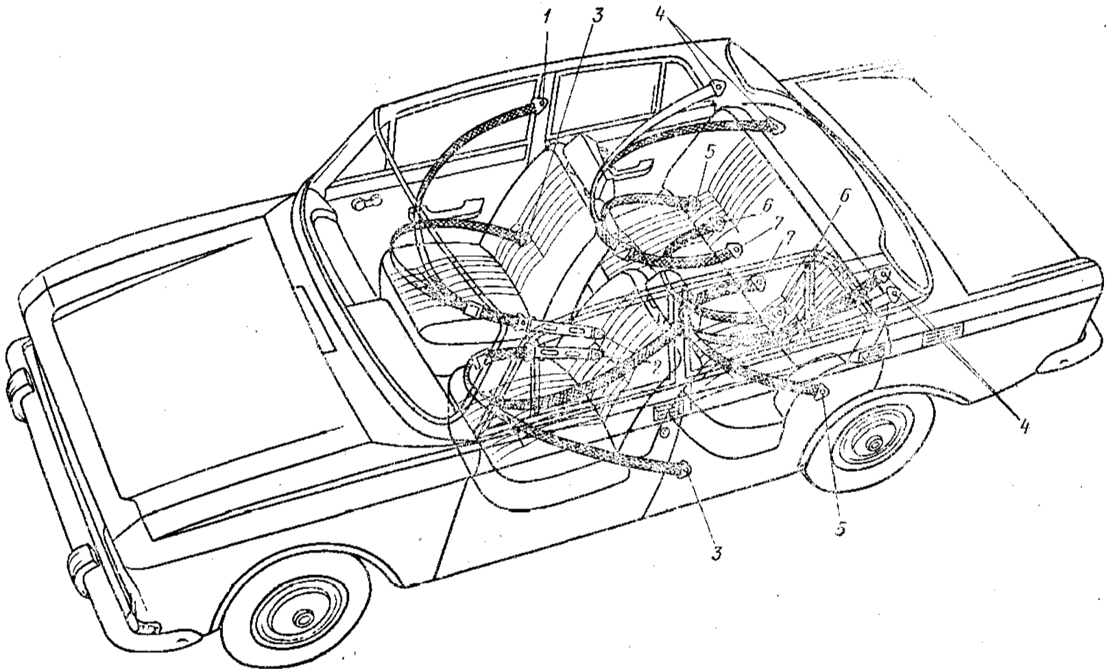
Рис. 19. Места крепления ремней безопасности
