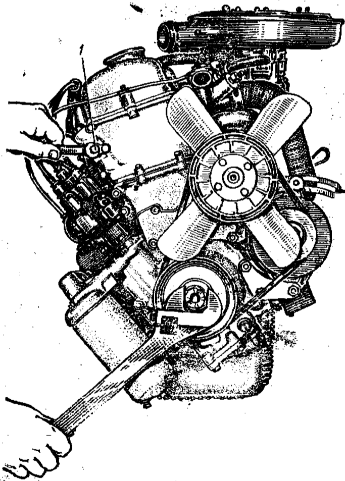
Рис. 53. Регулировка натяжения цепи привода газораспределения: 1 — стопорный болт
