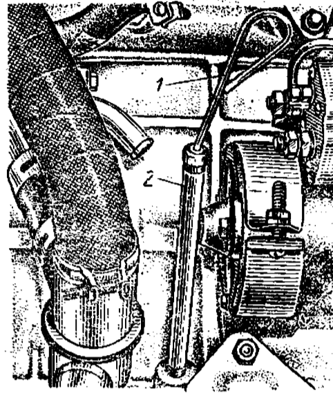
Рис. 43. Расположение маслoизмерительного стержня: 1 — стержень; 2 — направляющая трубка
