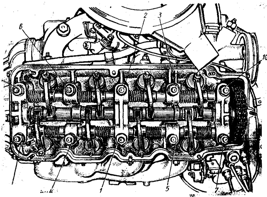
Рис. 54. Последовательность затяжки гаек шпилек, крепящих головку блока цилиндров к блоку
