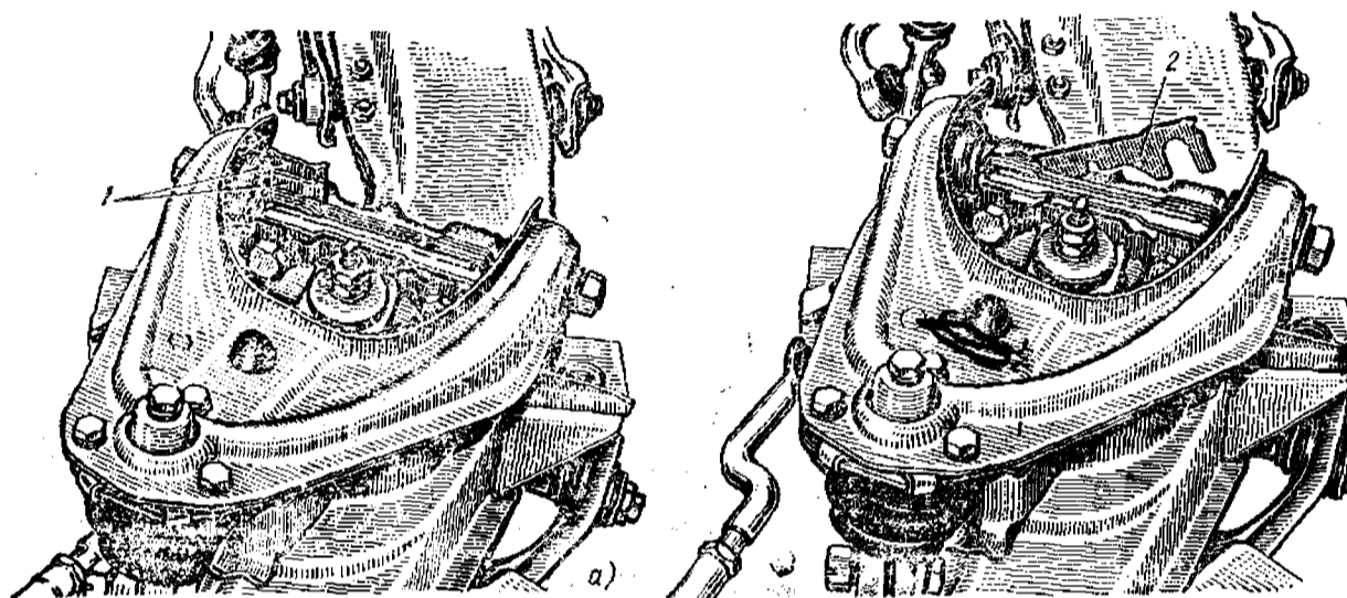
Рис. 69. Узел регулировки: а — угла продольного наклона поворотной стойки подвески; б — угла развала переднего колеса; 1 — регулировочные скобы; 2 — регулировочная прокладка
