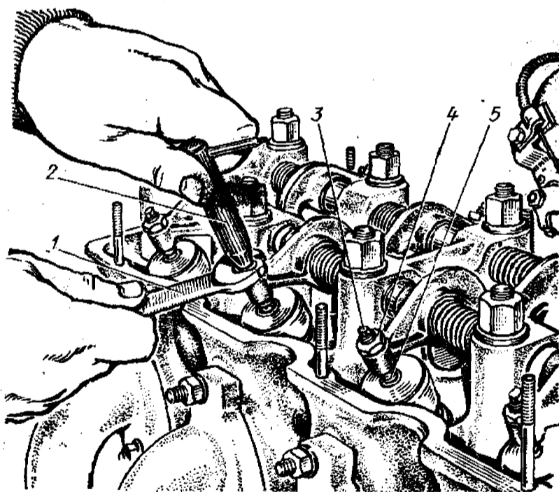
Рис. 52. Регулировка зазора между торцами наконечника и стержня клапана: 1 — рожковый ключ (14 мм); 2 — специальный торцовый ключ; 3 — нажимной болт; 4 — контргайка; 5 — наконечник
