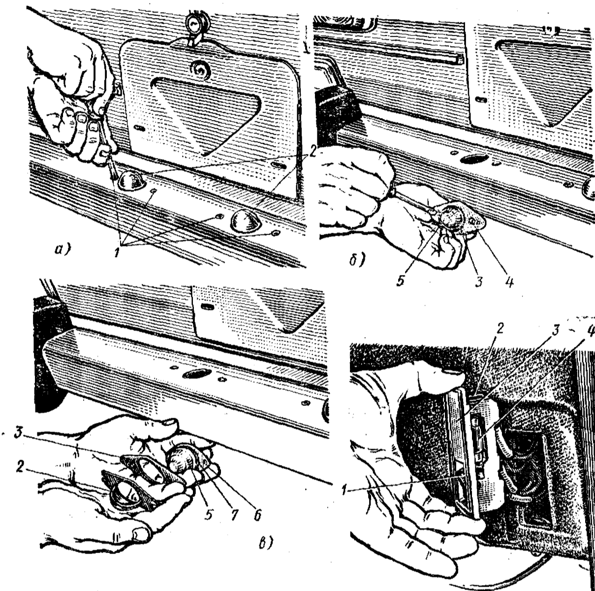
Рис. 95. Замена лампы в фонаре освещения номерного знака:
