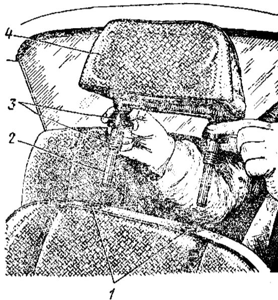
Рис. 18. Спинка сиденья со снятым подголовником: 1 — гнездо подголовника; 2 — штанга подголовника; 3 — ручка фиксатора; 4 — опорная поверхность подголовника
