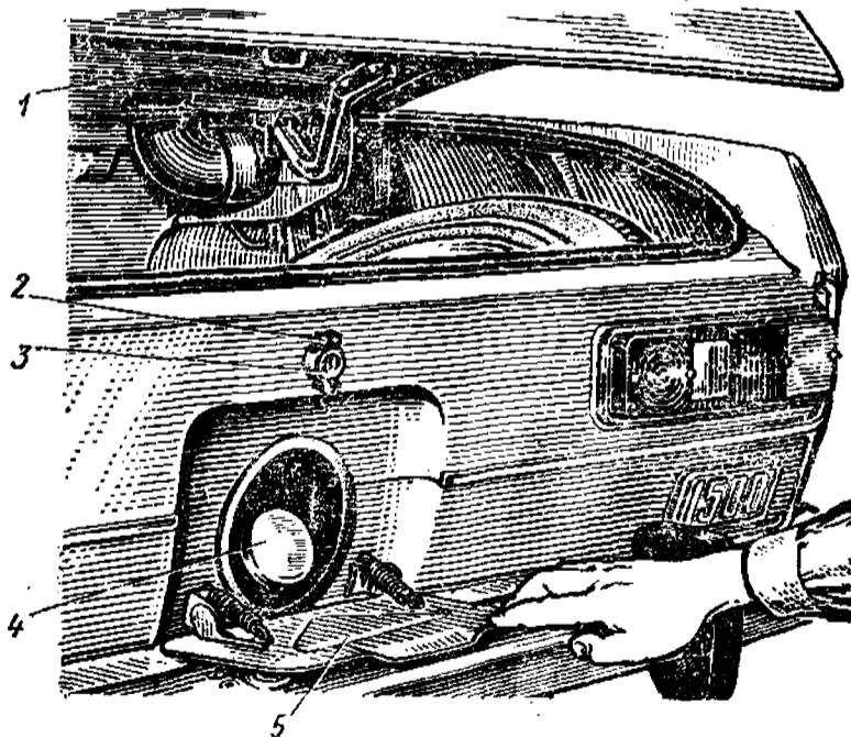
Рис. 15. Замок крышки багажника: 1 — защелка замка; 2 — ручка привода замка; 3 — цилиндр привода замка; 4 — пробка горловины топливного бака; 5 — крошштейн (крышка) измерного знака
