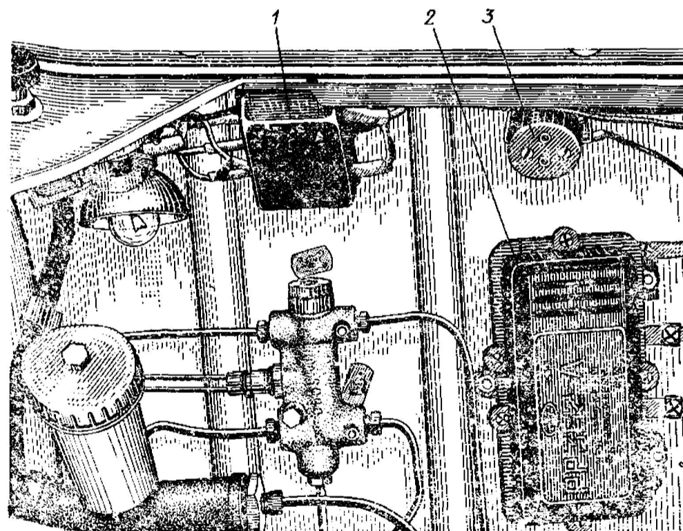
Рис. 82. Расположение реле-регулятора в подкапотном пространстве: 1 — блок плавких предохранителей; 2 — реле-регулятор; 3 — штексельная розетка для переносной лампы
