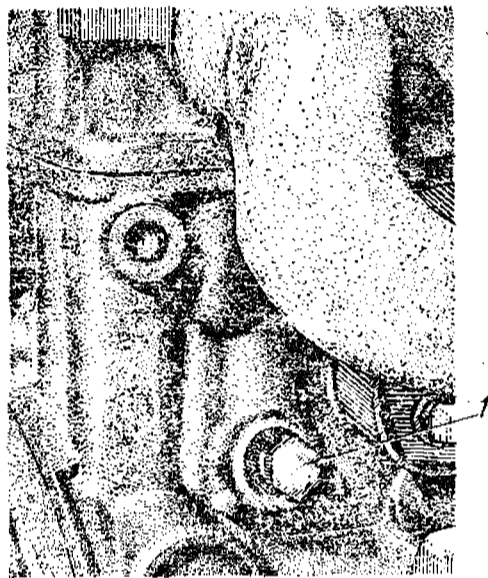
Рис. 38. Расположение пробки сливного отверстия на стенке рубанки блока цилиндров: 1 — пробка
