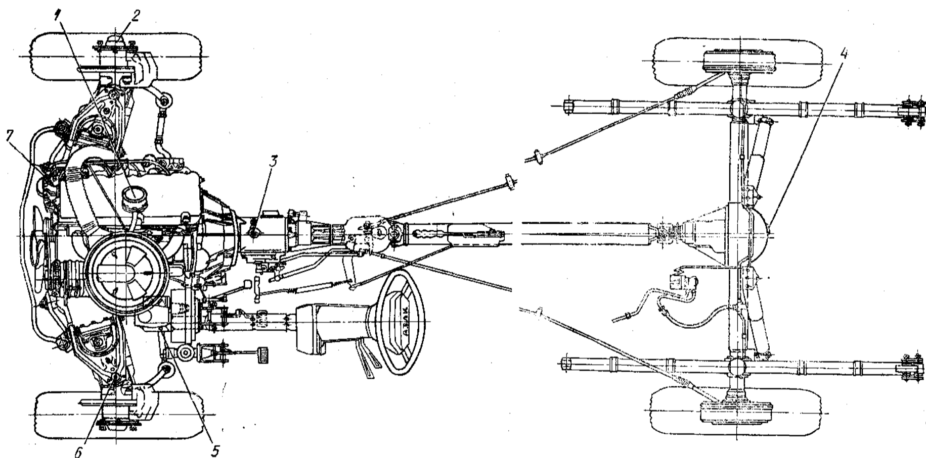
Рис. 41. Карта смазки агрегатов, узлов и механизмов шасси автомобиля (обозначение позиций см. табл. 3)
