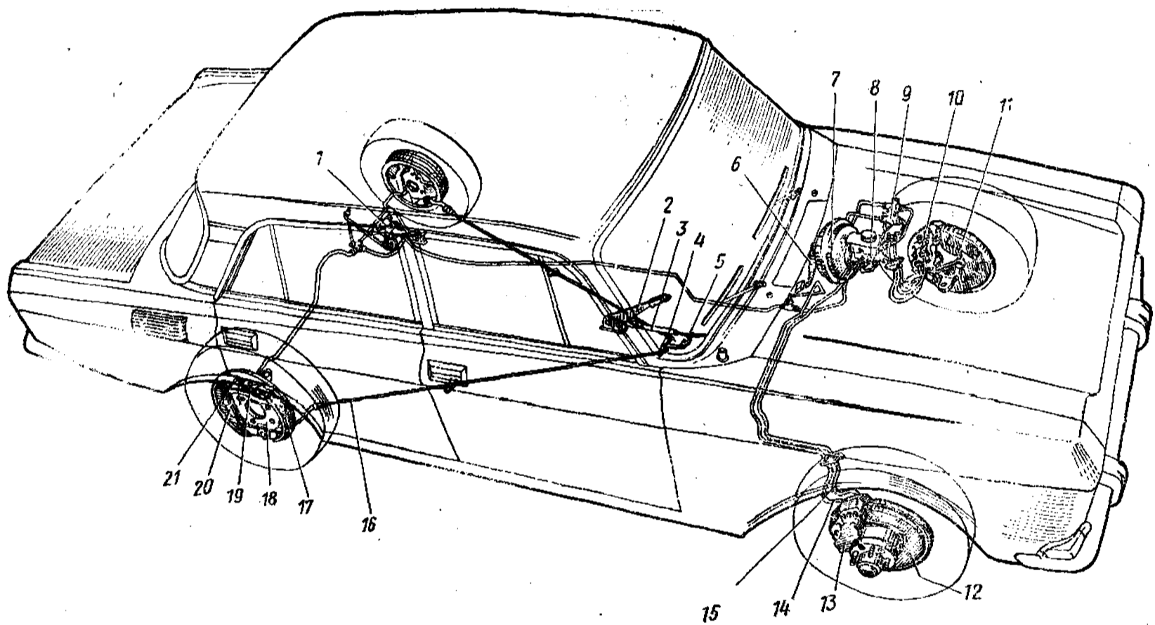
Рис. 74. Схема тормозных систем:
